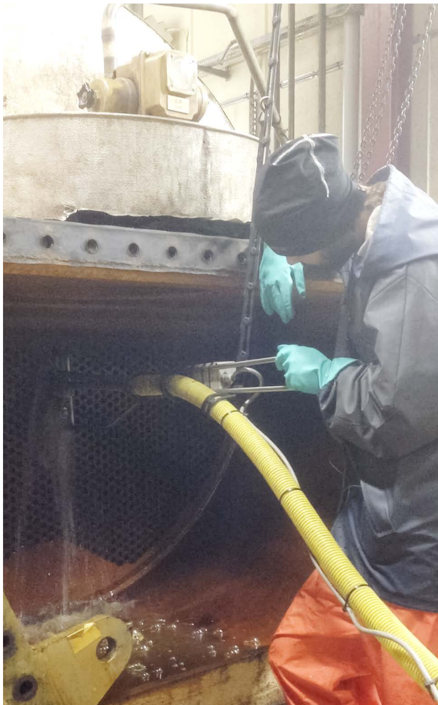
Tvätt av stora värmväxlare i samarbete med Vattenfall. Operatören fäster munstycket från roboten i hålen som ska tvättas. Därefter sker tvätt med iller som matas ut automatiskt i jämn hastighet. Operatören slipper bli nersmutsad av tvättvatten och tvättresultatet blir jämnare och bättre.
